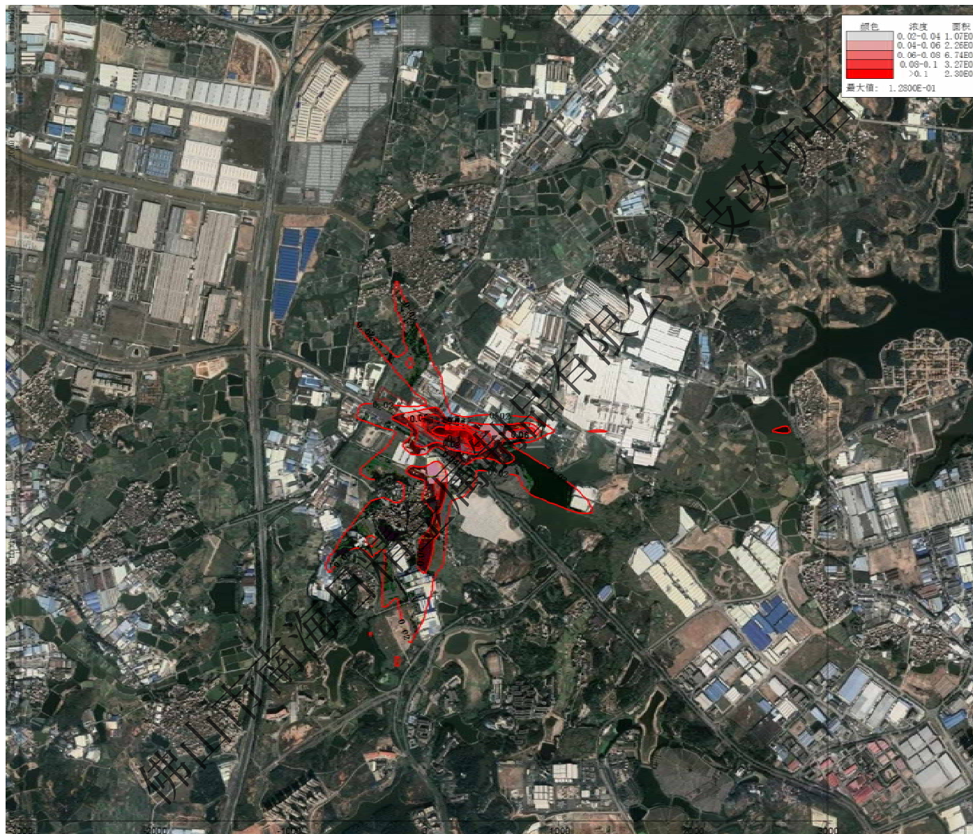
图5.3-18 正常排放时，硫酸雾1小时平均浓度贡献值等值线图
