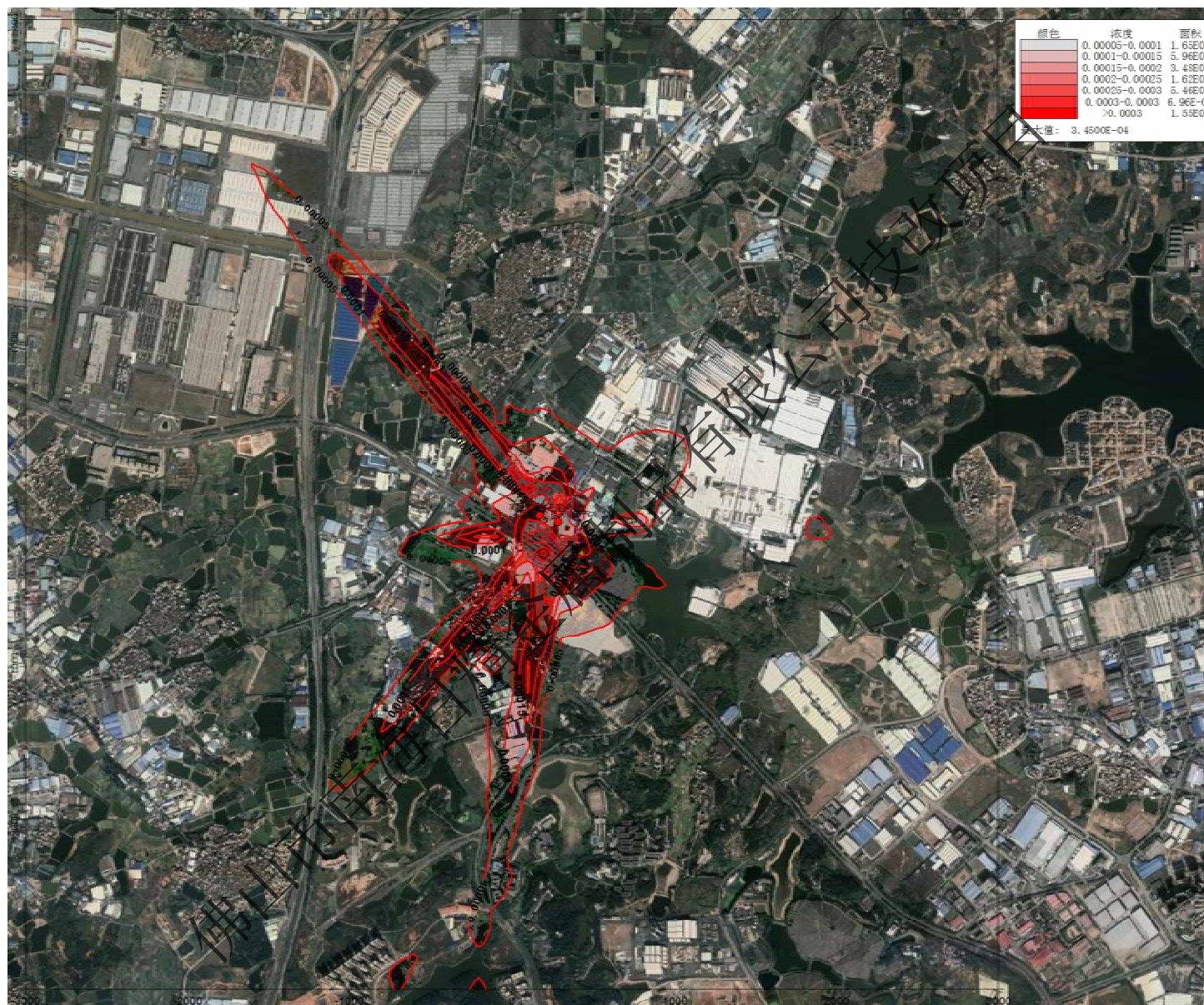
图5.3-21 正常排放时，氟化物1小时平均浓度贡献值等值线图
