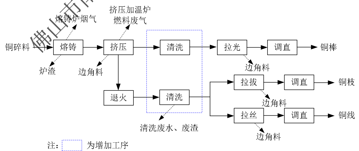
图 3.2-1 技改后铜棒、铜枝、铜线生产工艺流程图
