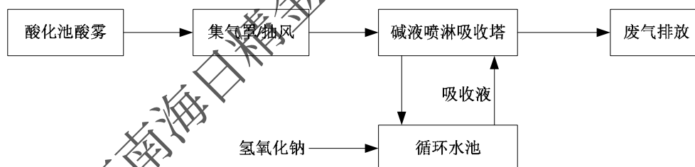
图 6.2-1 酸雾处理工艺流程图
