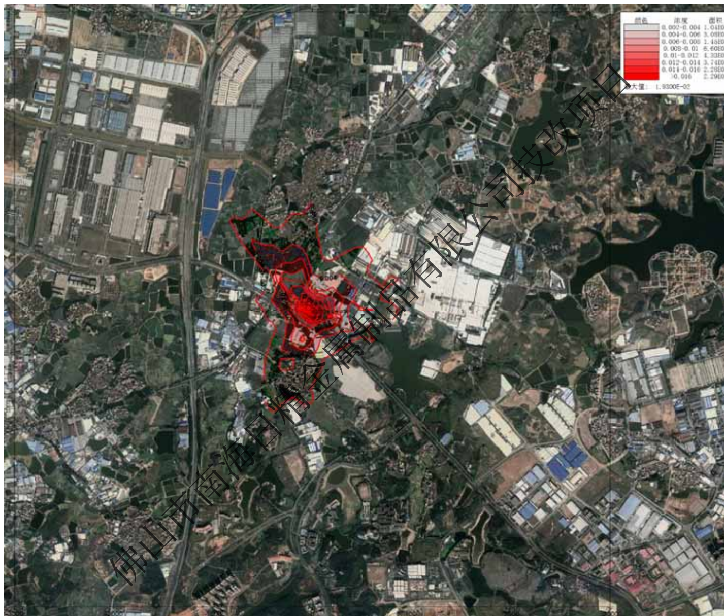
图5.3-16 正常排放时，TSP日平均浓度贡献值等值线图
