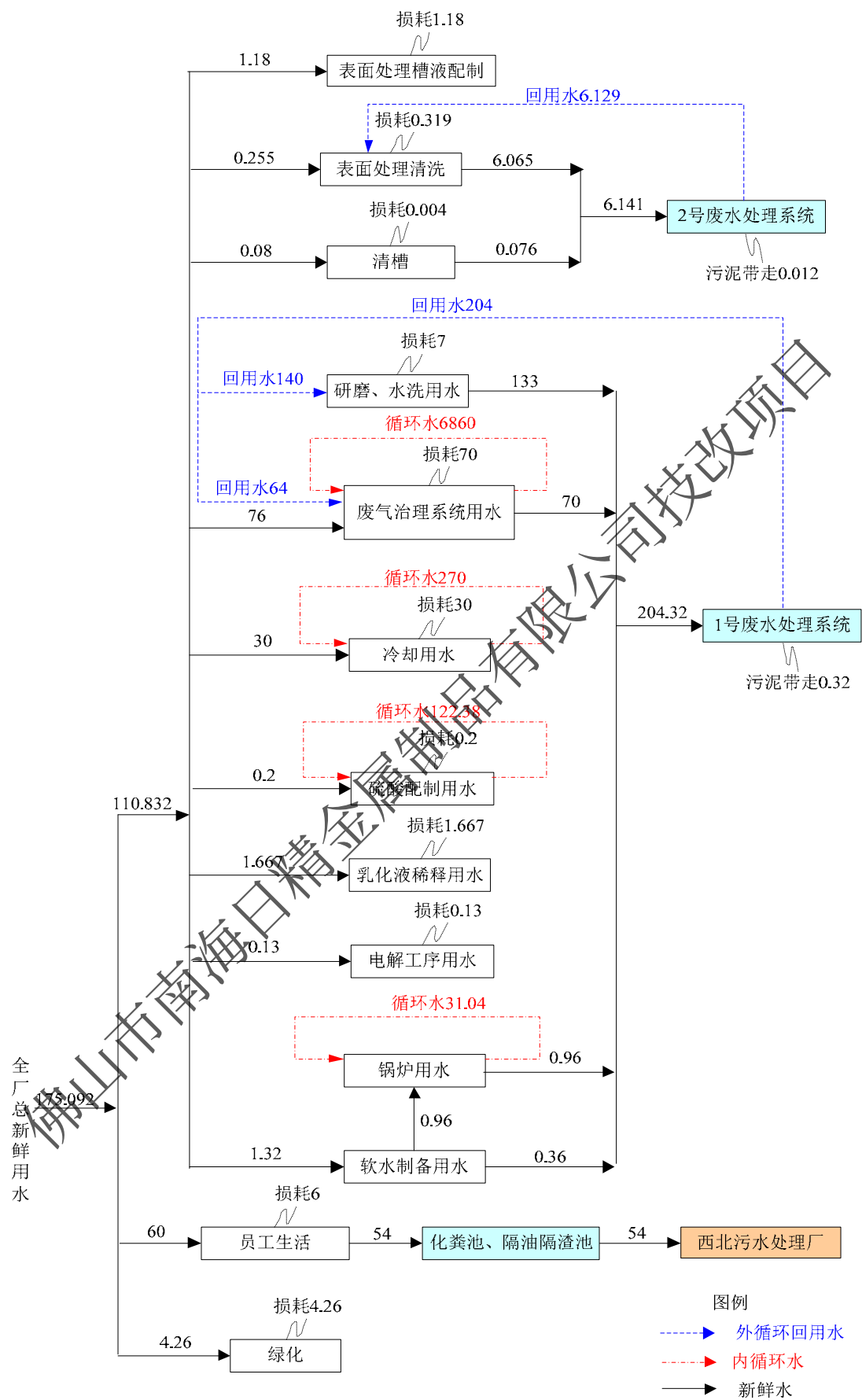
图 3.3-6 本项目给排水平衡图（单位：m³/d）
