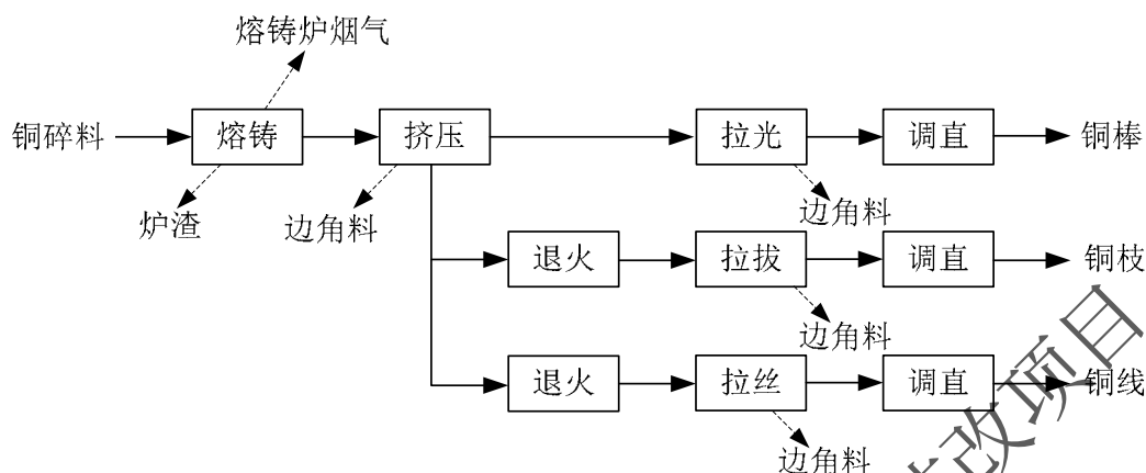
图 2.3-1 原有项目铜棒、铜枝、铜线生产工艺流程图
