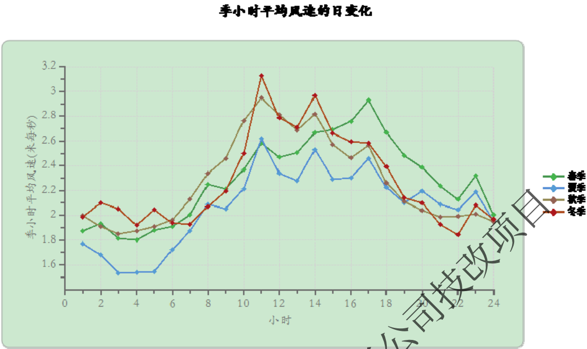
图5.3-3 2016年各季小时平均风速日变化曲线图
