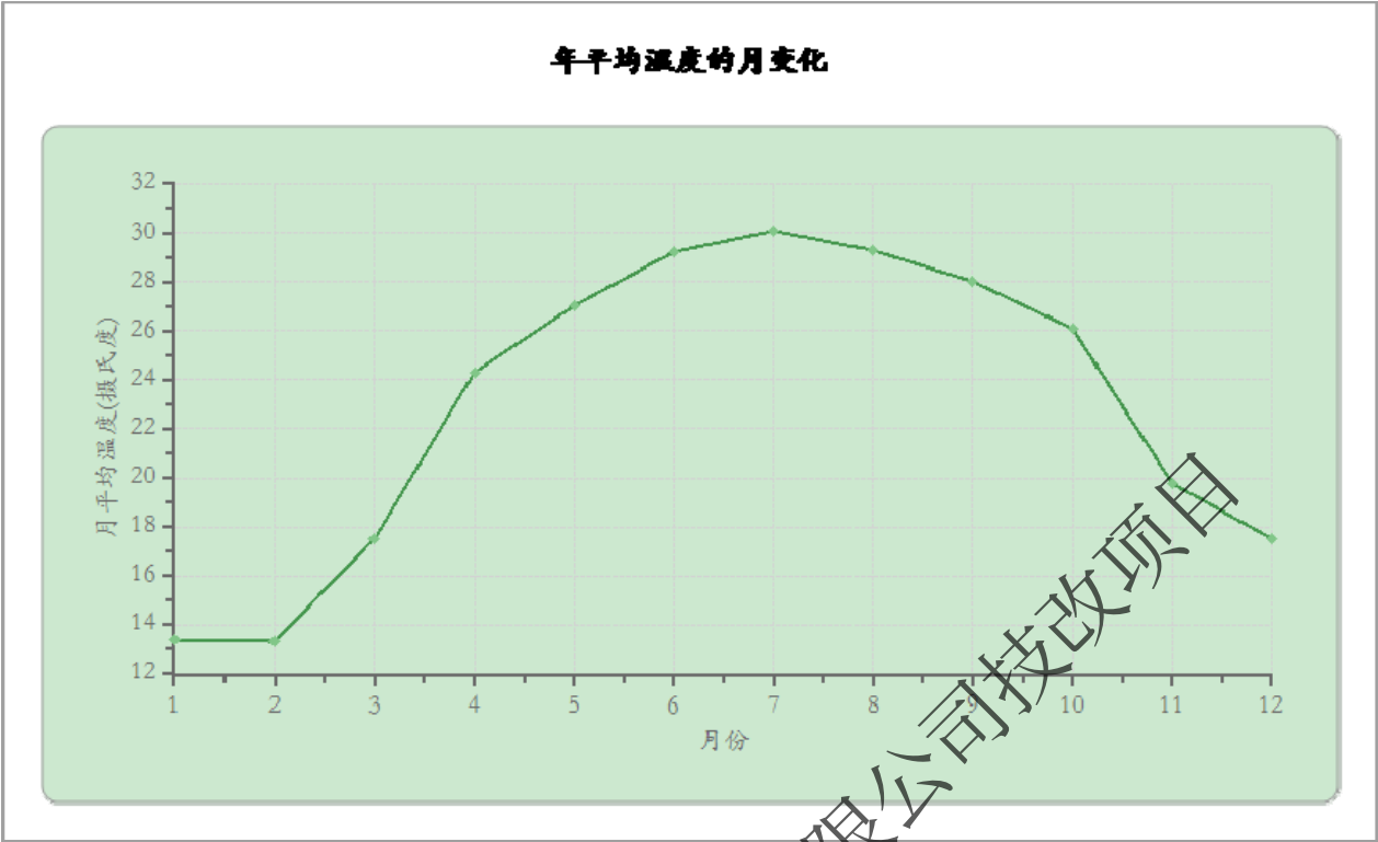
图 5.3-1 2016 年平均温度月变化曲线图
