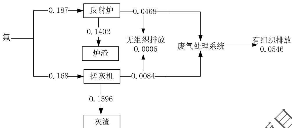
图 2.4-4 原有项目氟元素平衡图（单位：t/a）
