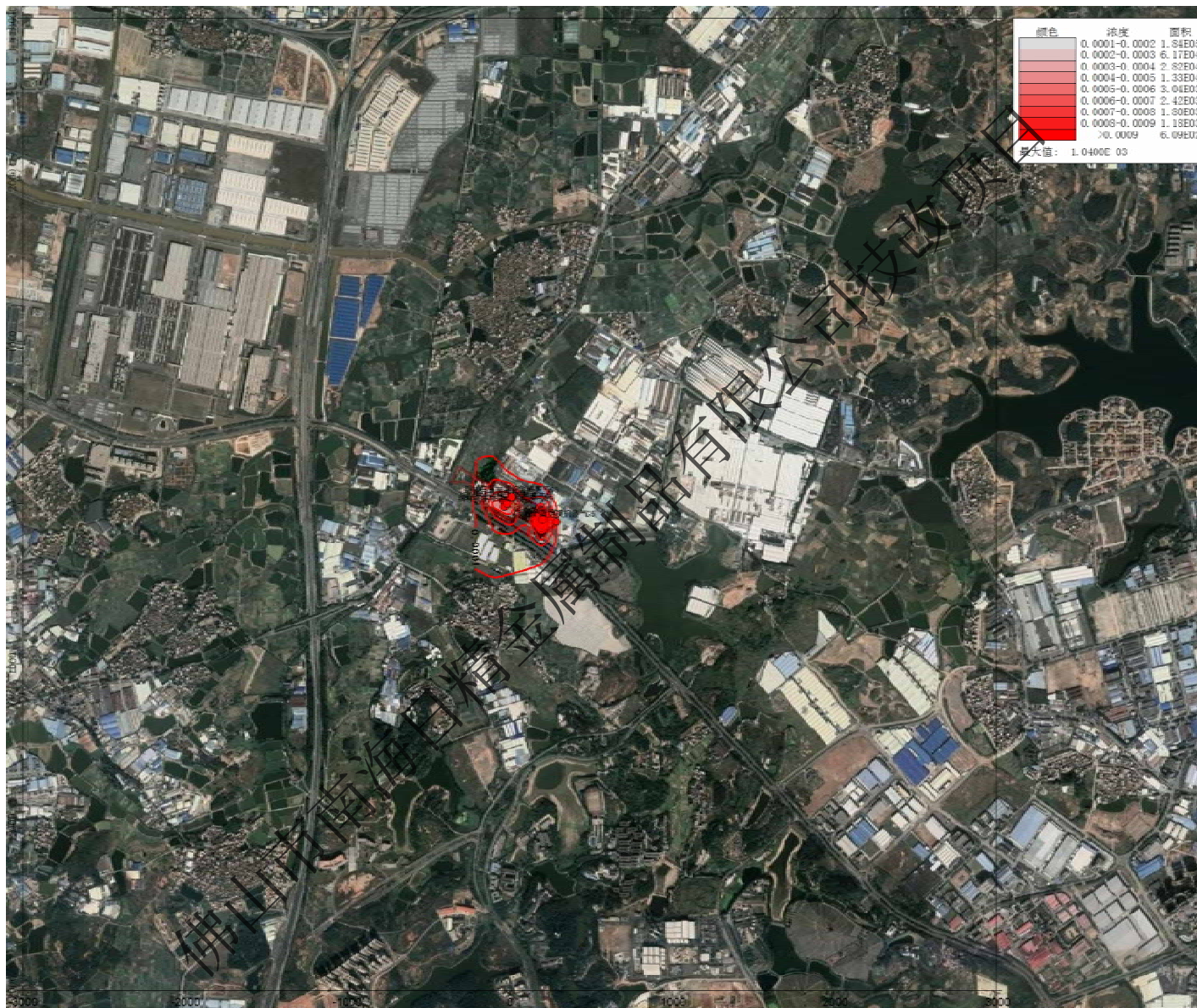
图5.3-8 正常排放时，SO 2 年平均浓度贡献值等值线图
