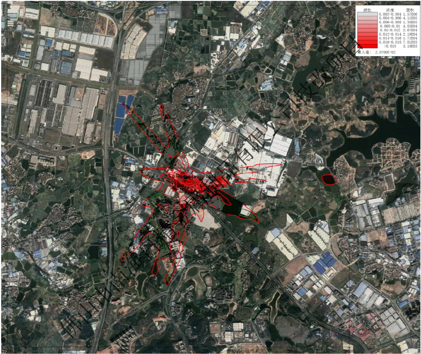
图5.3-19 正常排放时，硫酸雾日平均浓度贡献值等值线图
