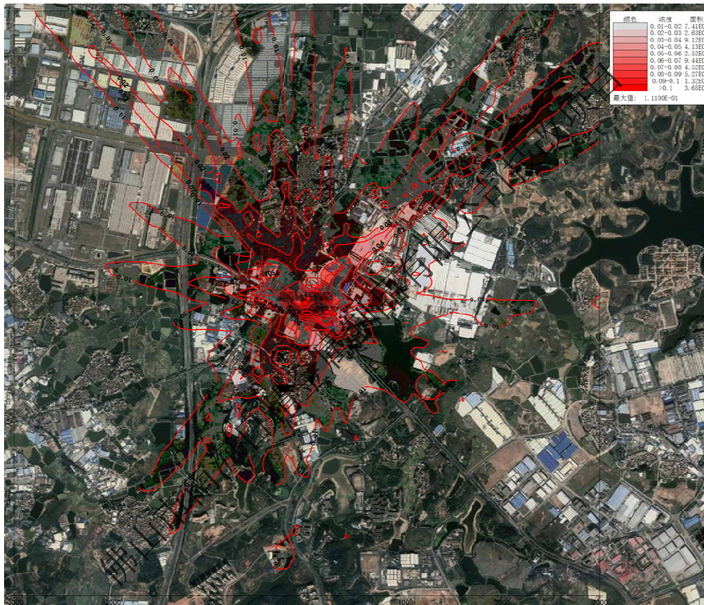
图5.3-9 正常排放时，NO x 1小时平均浓度贡献值等值线图
