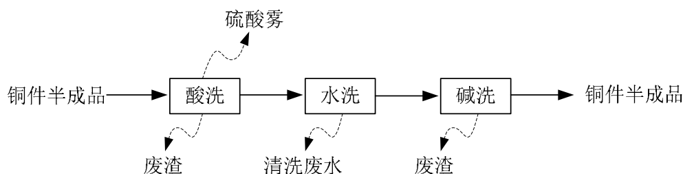
图 3.2-2 技改后清洗工艺流程图
