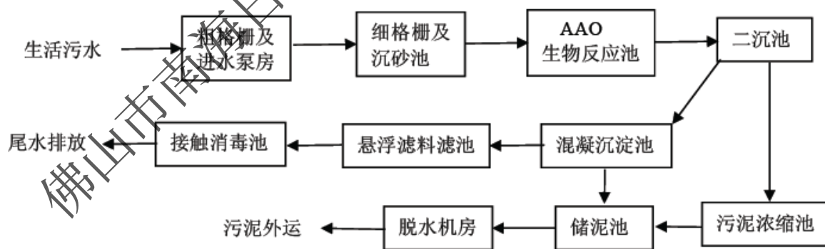
图 5.2-1 西北污水处理厂工艺流程图
