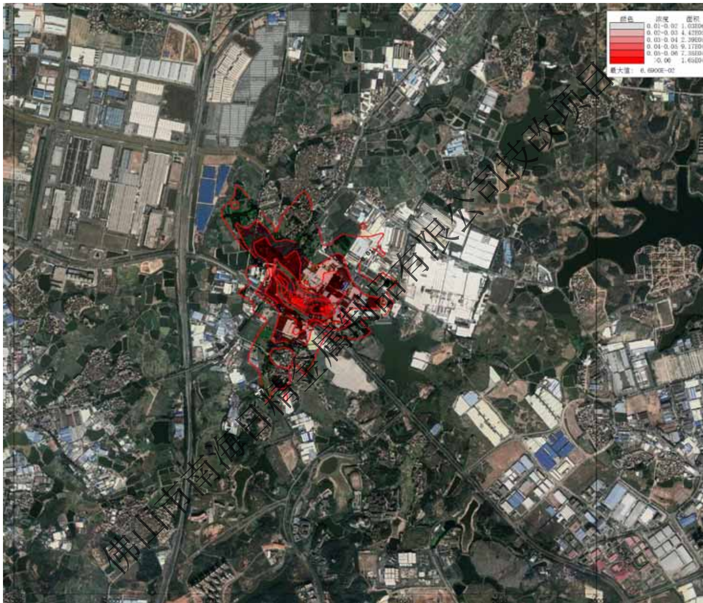
图5.3-15 正常排放时，TSP1小时平均浓度贡献值等值线图
