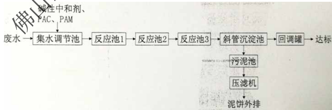
图 3.5-1 工业废水处理系统工艺流程图
