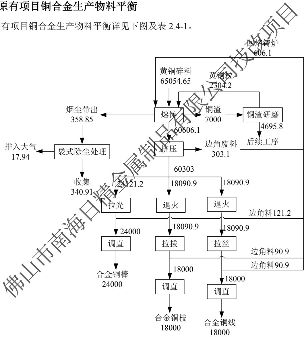
图 2.4-1 原有项目铜合金生产物料平衡图（单位：t/a）
