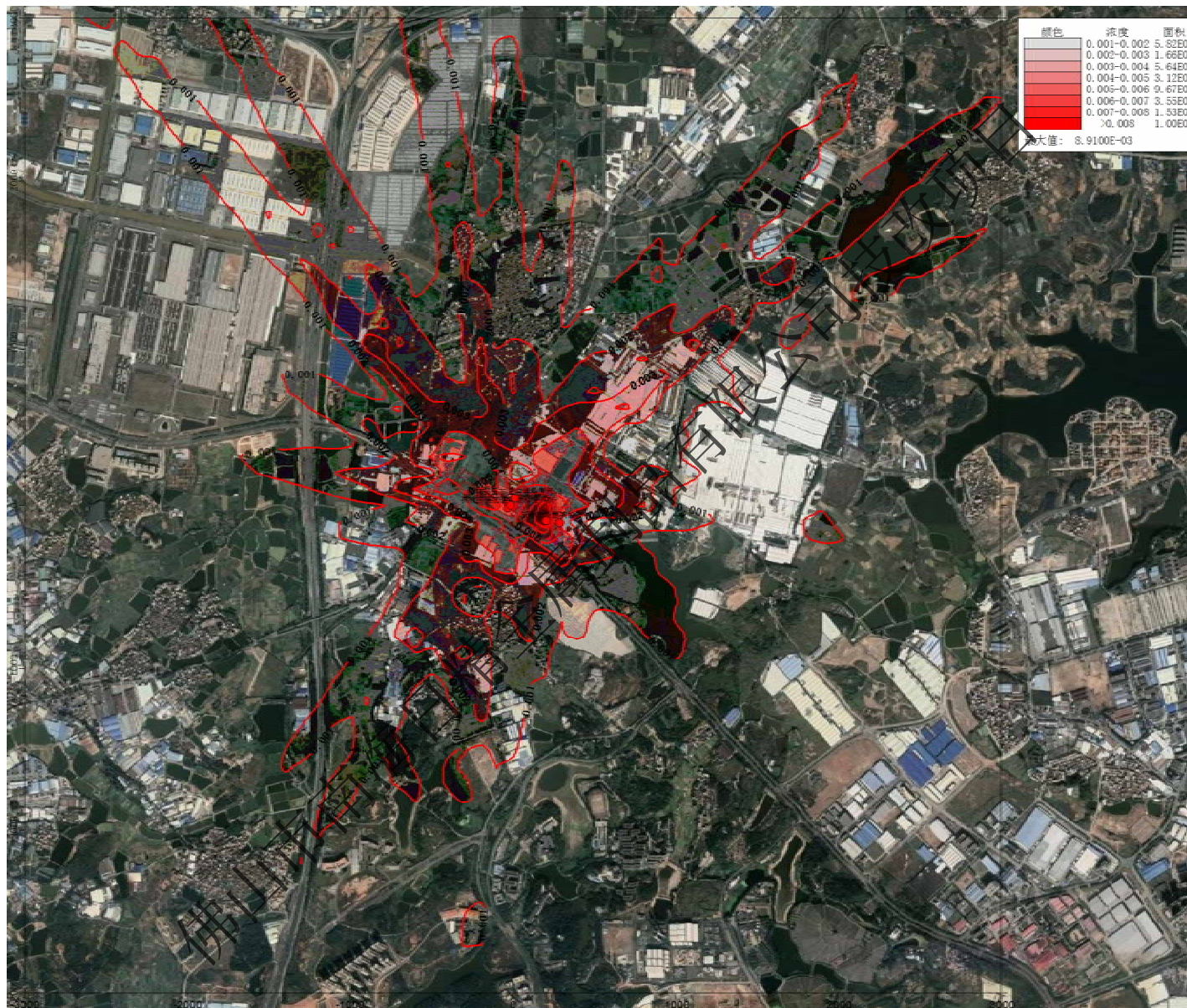
图5.3-6 正常排放时，SO 2 1小时平均浓度贡献值等值线图
